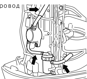
Топливопровод
