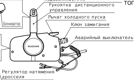
УЗЕЛ ДИСТАНЦИОННОГО УПРАВЛЕНИЯ
