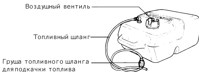
ТОПЛИВНЫЙ БАК
